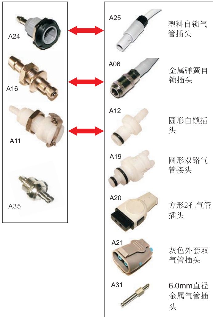
仪器端插座
